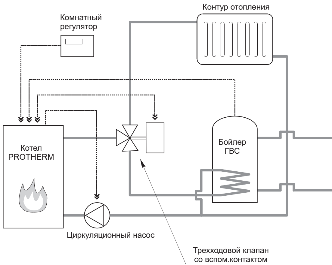
Рис.4 Схематическое изображение "совместной работы" котла с внешним бойлером и установка насоса
