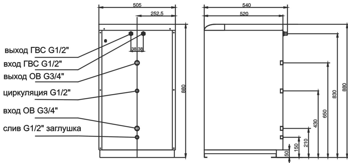
Рис. 1 Основные и соединительные размеры
