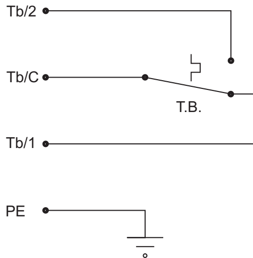
Рис.2 Схема электрического подключения бойлера PROTHERM В 100
